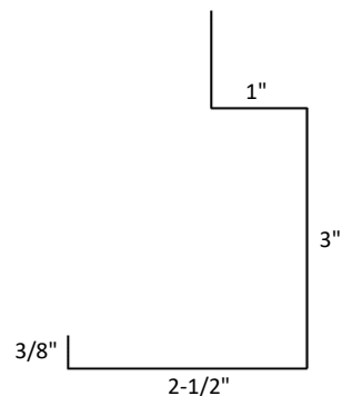
Sliding Door Trim
